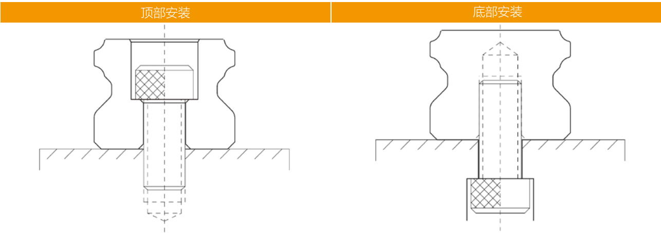
(1) 底部安装导轨尺寸图
