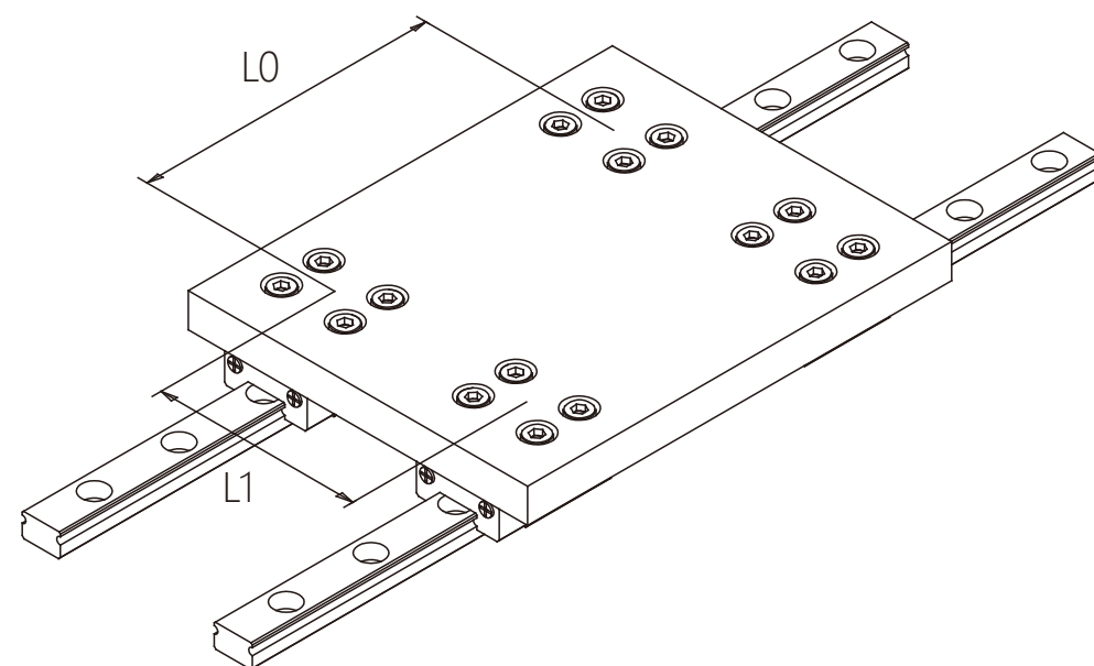
跨距尺寸示意图
