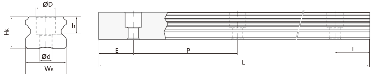
(2) 大型安装孔-顶部安装导轨尺寸图
