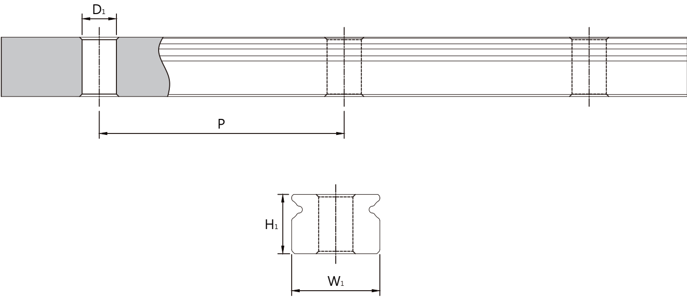
下锁式尺寸图
