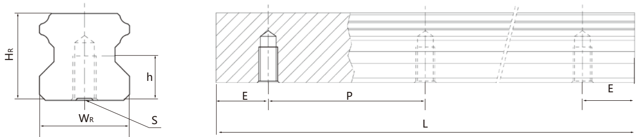
(1) 底部安装导轨尺寸图
