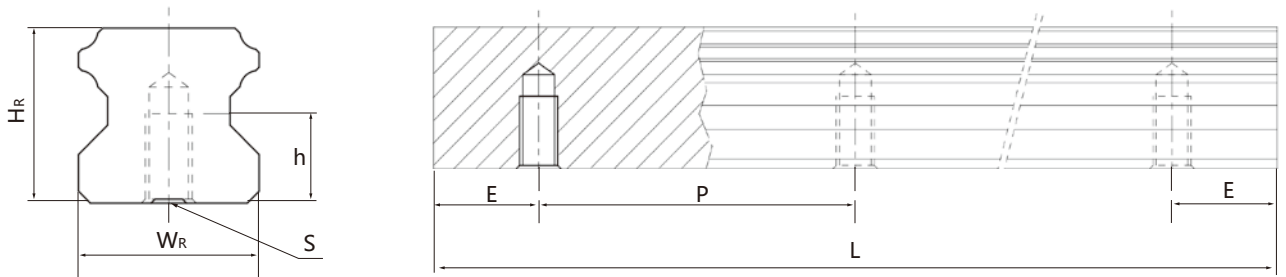
(1) 底部安装导轨尺寸图
